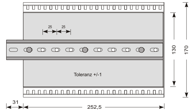
Montageteil M 250 (ES/DS) ABB. 2
