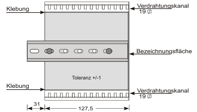
Montageteil M 125 (ES/DS)
